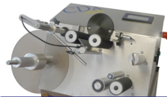
angetriebenes Drei-Rollen-System
